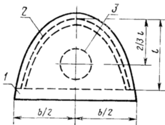
1—верх обуви; 2—жесткий носок; 3—место установки пластилинового столбика. l —длина носка; b —максимальная ширина носковой части
