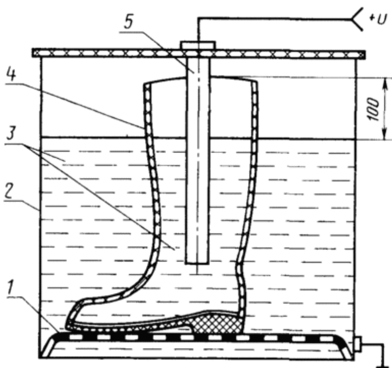
1—сетка; 2—ванна; 3—электролит; 4—образец; 5—электрод
