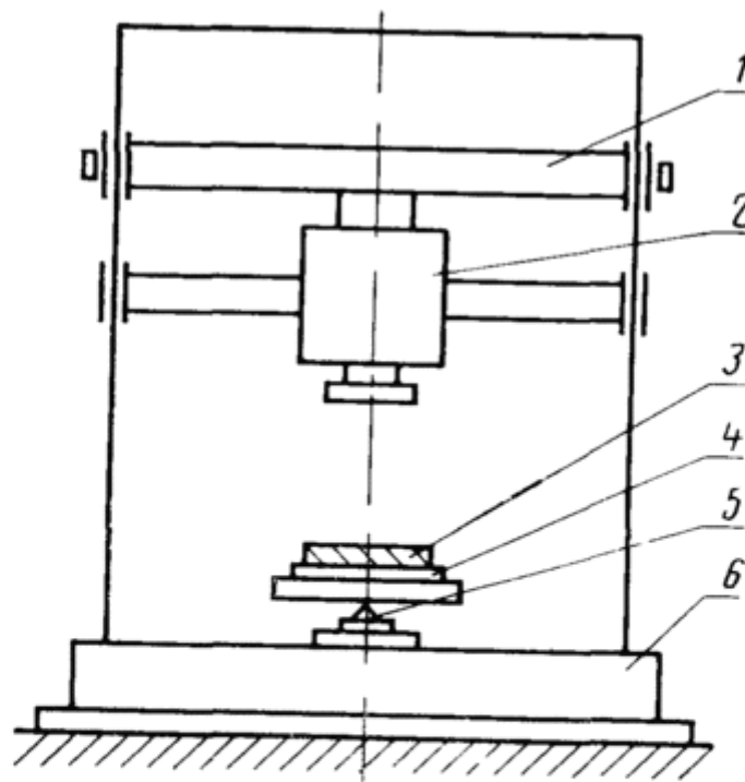
1- каретка; 2-боек; 3-защитный элемент; 4-плата; 5-датчик; 6-основание
