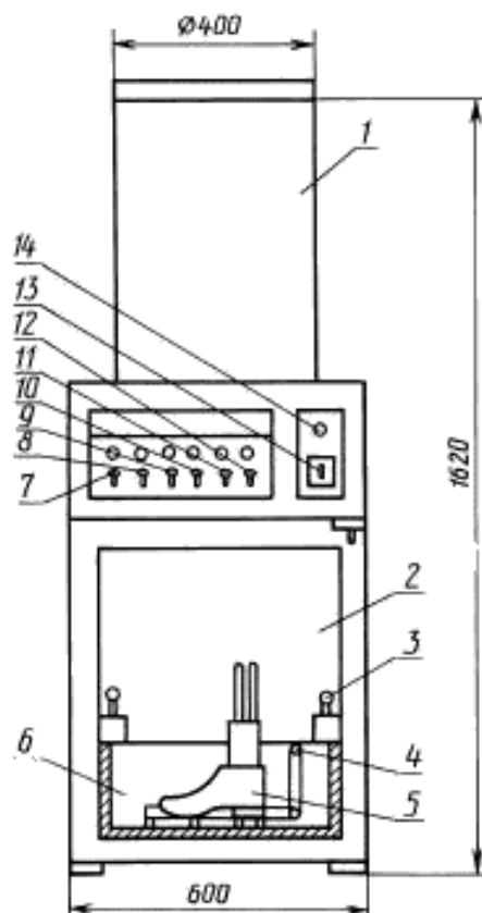
Прибор для определения пылепроницаемости спецобуви ЭПОП
