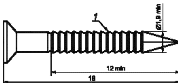
1 — не менее 13 полностью сформированных упорных кромок
